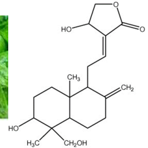
สารแอนโดรกราโฟไลด์ (andrographolide)
